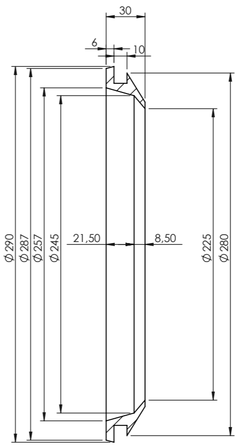
SEZIONE E-E
